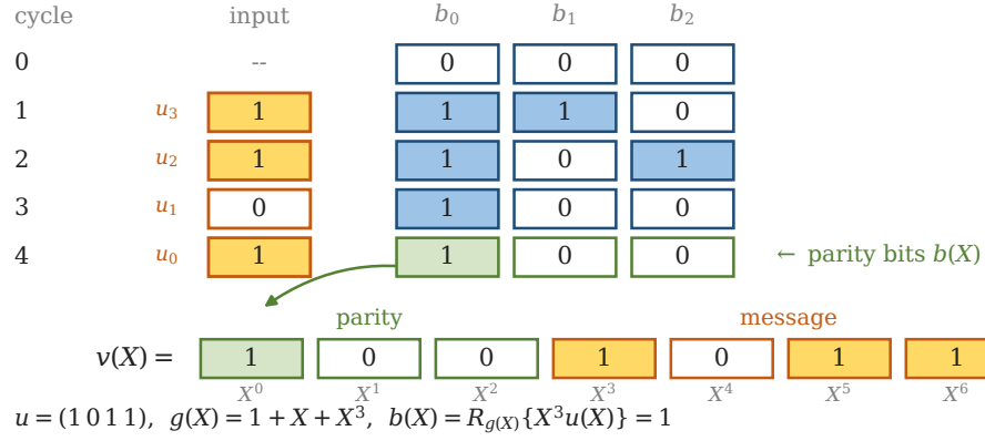
Figura 4: Traza del codificador sistemático del código (7,4) para el mensaje \mathbf{u} = (1\ 0\ 1\ 1) . Los bits ingresan empezando por u_3 ; al cabo de k = 4 ciclos el registro contiene la paridad \mathbf{b} = (1\ 0\ 0) , que se antepone al mensaje para formar la palabra transmitida. Los valores reproducen el Ejemplo 5.5 de Lin & Costello, Error Control Coding , 2ª ed.
